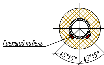
Монтаж двух ниток греющего кабеля
