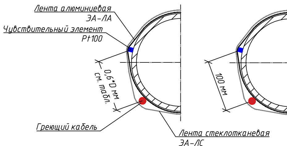
Рисунок 6.2– Установка чувствительного элемента на трубопровод
