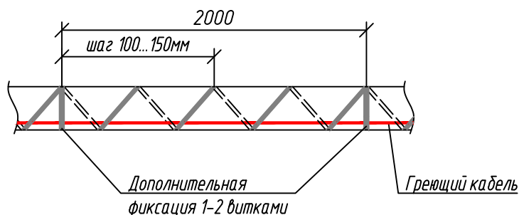
Рисунок 5.9.6 – Крепление греющего кабеля
