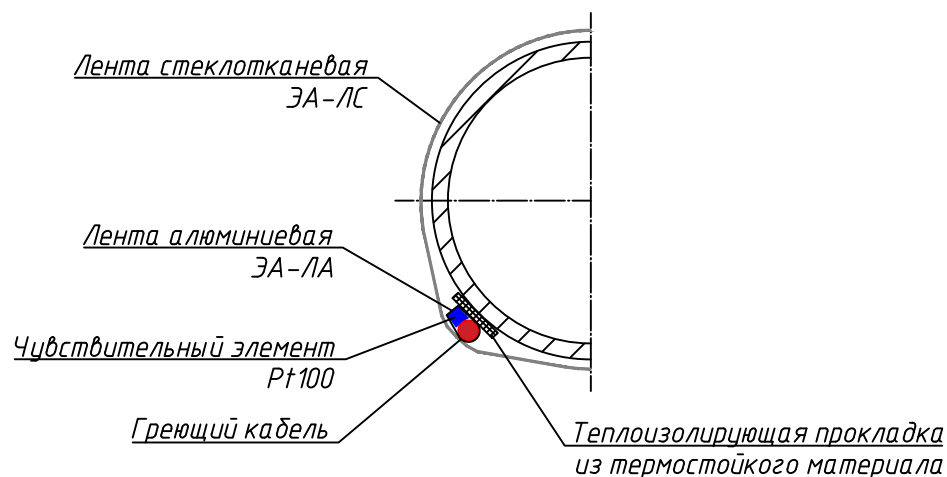
Рисунок 6.3 – Установка чувствительного элемента на поверхность греющего кабеля (в случае необходимости контроля температуры греющего кабеля)
