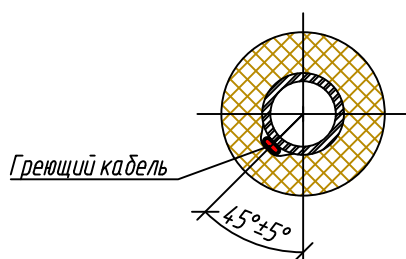
Монтаж одной нитки греющего кабеля
